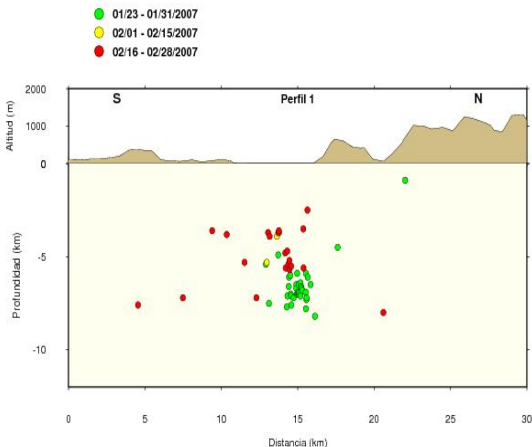
Fig. 2 Perfil en profundidad que cruza el fiordo Aysén de acuerdo a la línea roja presentada en la Fig. 1.
